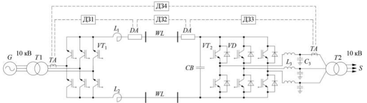
4.2 – сурет-Қорғаныс бөлімдері бар тұрақты ток беру
