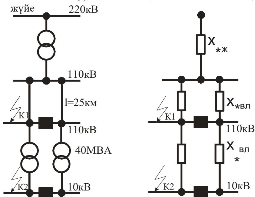
2.5-сурет-Электрмен жабдықтаудың алмастыру сұлбасы
