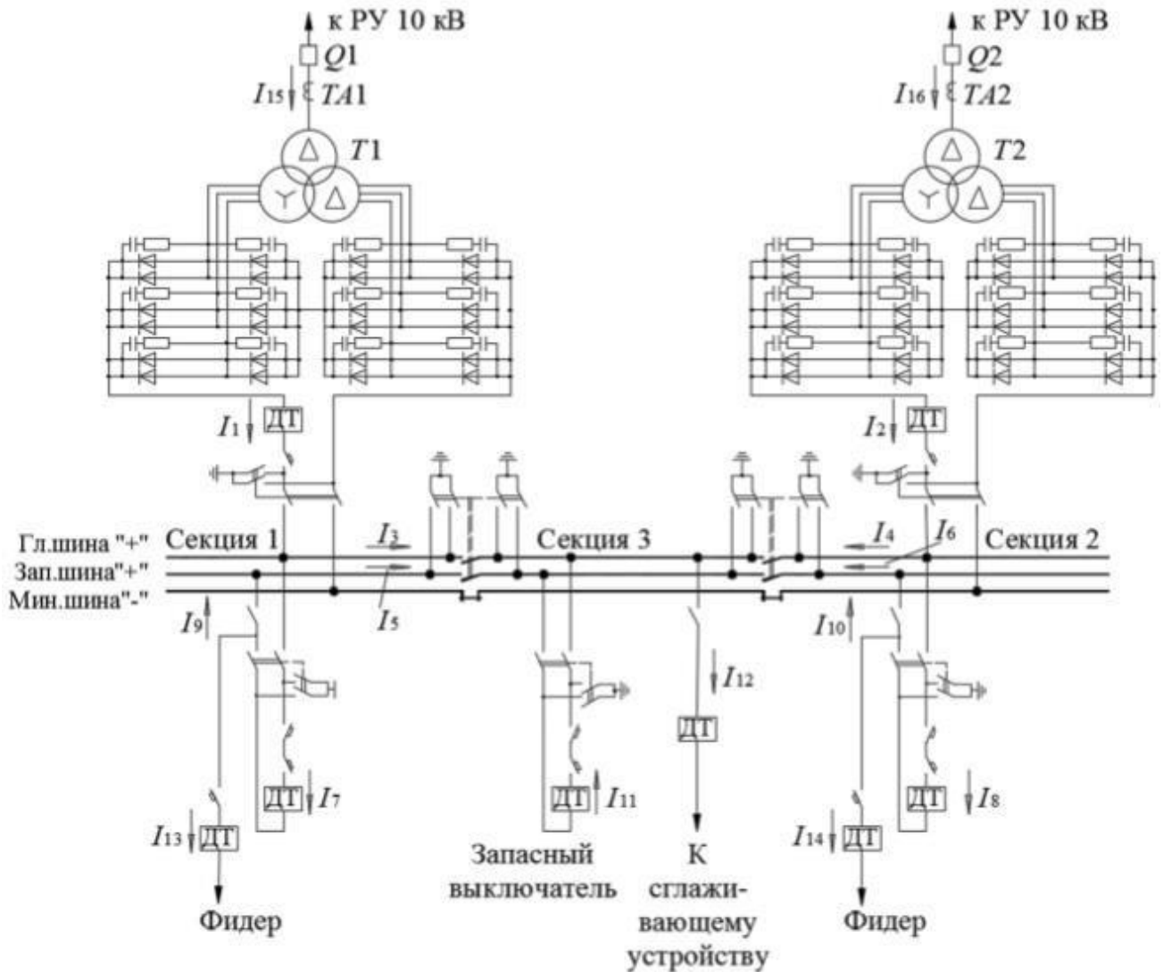
4.6 – сурет-3,3 кВ тарту құрылғысының сұлбасы
